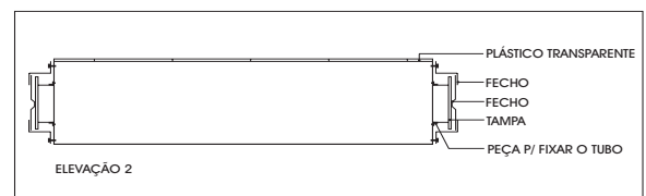
Figura 2. Esquema para construção do coletor solar.
